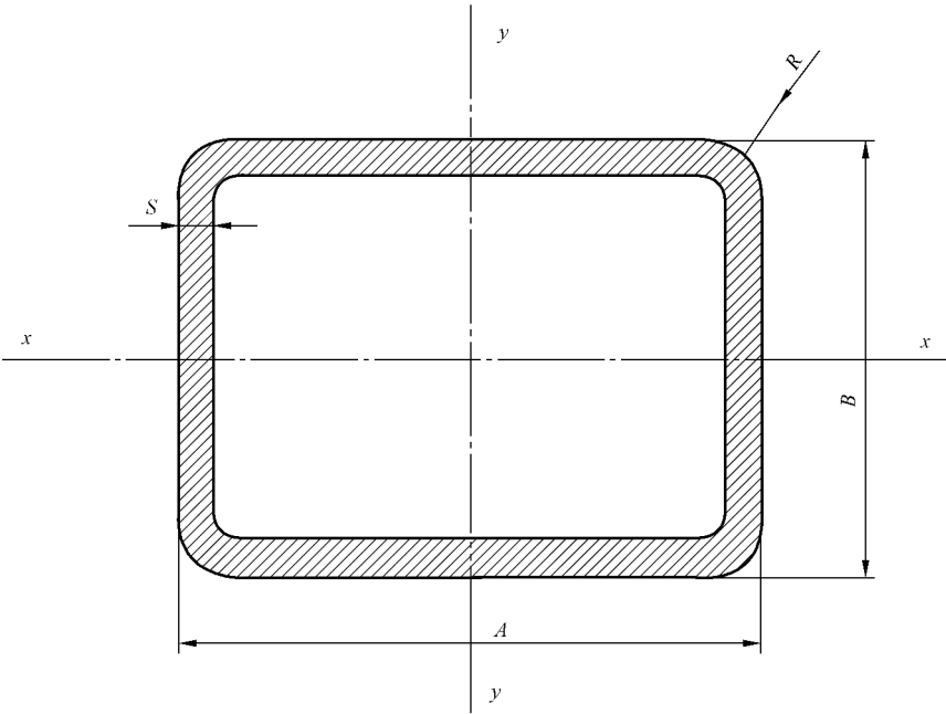
图 A.2 矩形钢管 (D-2)
