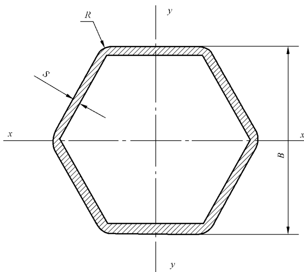
图 A.5 内外六角形钢管(D-5)
