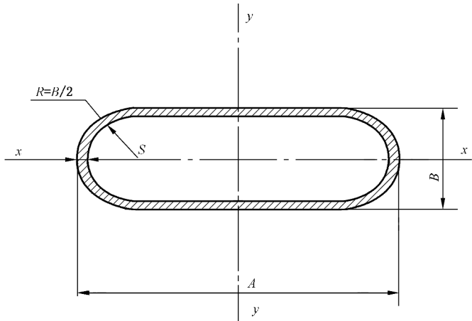
图 A.4 平椭圆形钢管(D-4)
