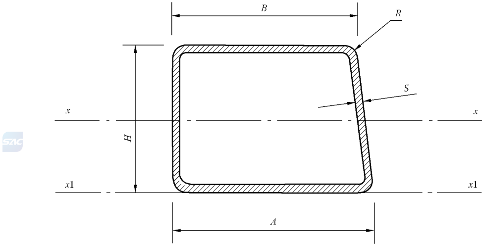
图 A.6 直角梯形钢管(D-6)
