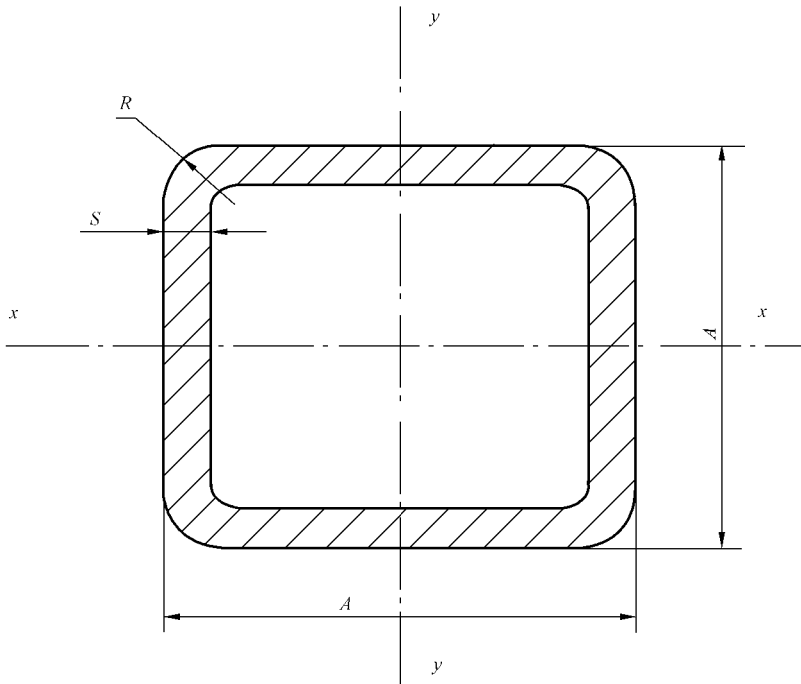
图 A.1 方形钢管(D-1)
