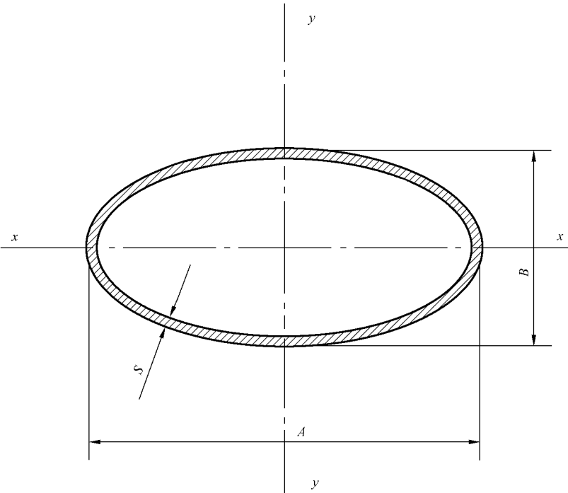
图 A.3 椭圆形钢管(D-3)
